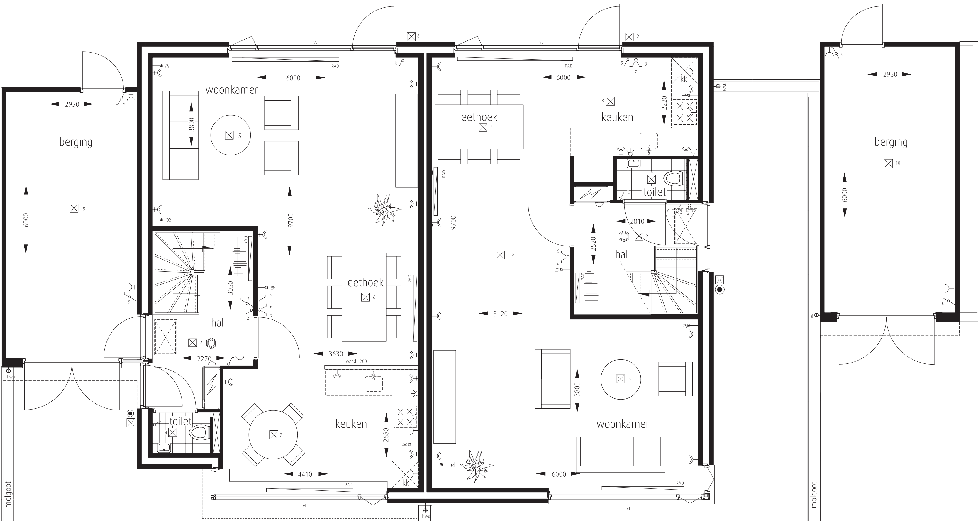
begane grond [schaal 1:50] bouwnummers 34-38 en 29-31-35 gespiegeld
