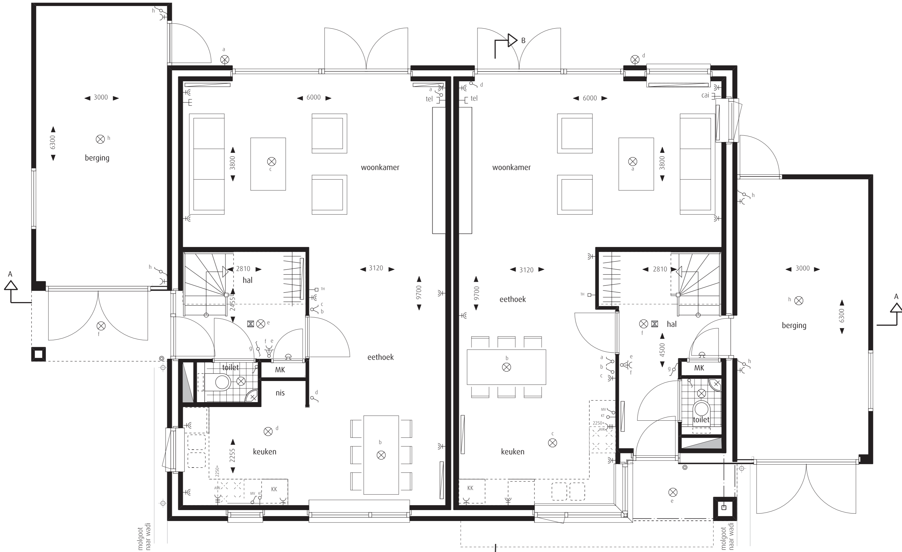
begane grond [schaal 1:50] bouwnummers 20-24-28
