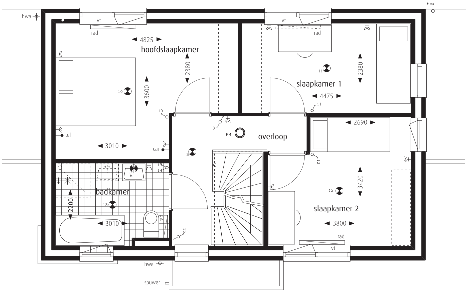
Berkenhaege 1e verdieping [schaal 1:50] kavelnummer 16B
